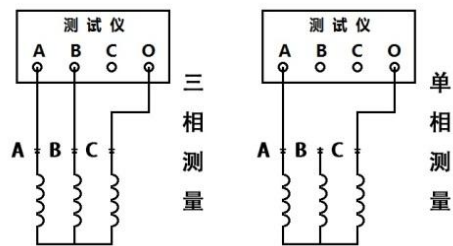
接线方式：Y型
