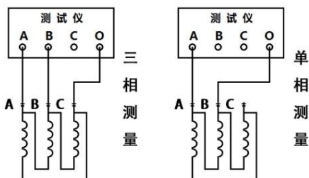
接线方式：△型
