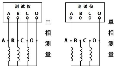
接线方式：YN型
