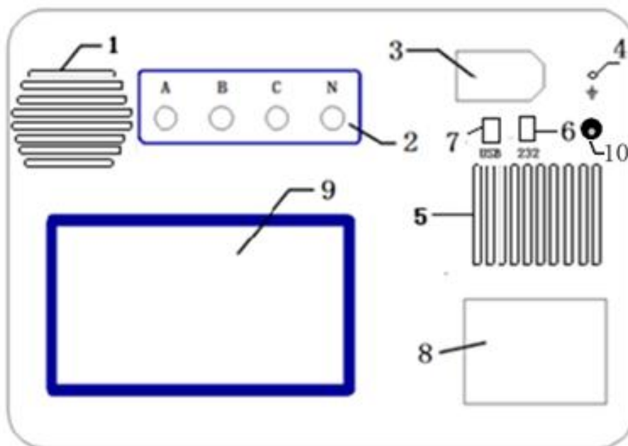
图 5.1 面板图
